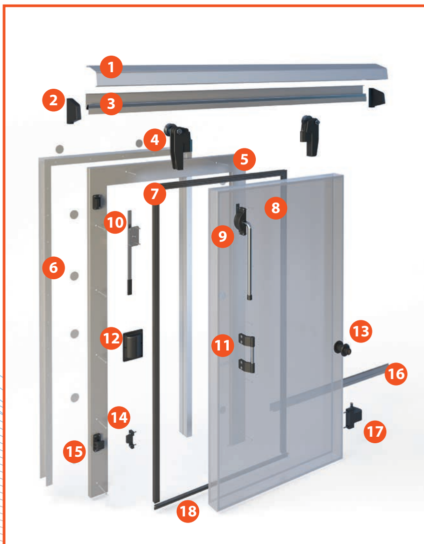
Рисунок 1. Откатная холодильная дверь
