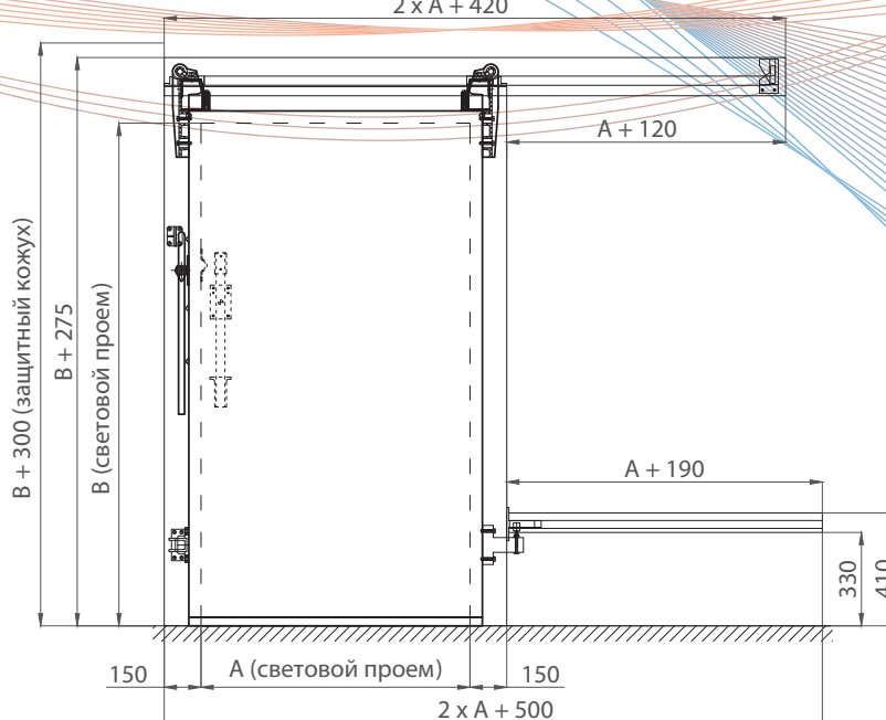
Рисунок 2. Откатная холодильная дверь 2 \times A + 420
